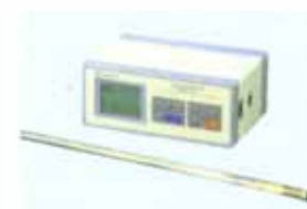
中高温風速計 (MODEL6162) 500℃までの風速を測定 日本カノマックス(株)製品使用
